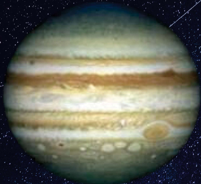
木星
