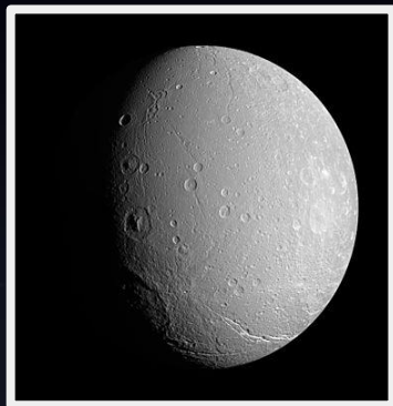
土衛四
