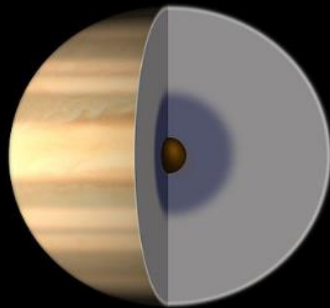
土星
