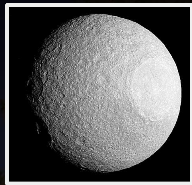
土衛三
