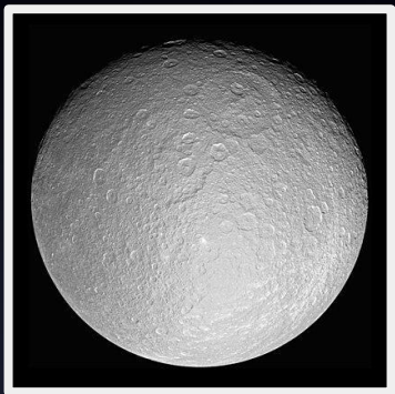
土衛五
