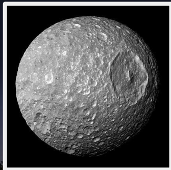
土衛一
