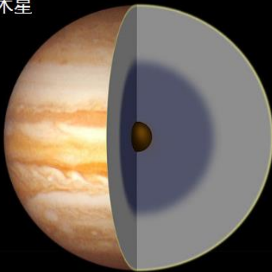
木星
