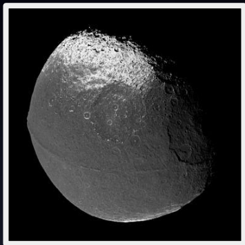
土衛八
