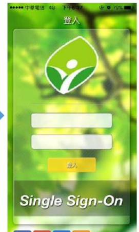
圖 2 帳密輸入頁
